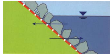
Protección filtro
